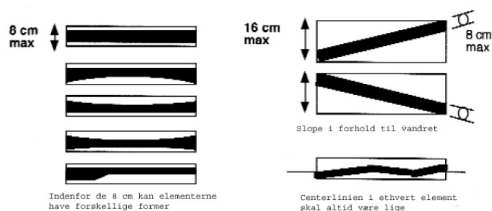
Figur 4 Elementernes dimensioner 2
