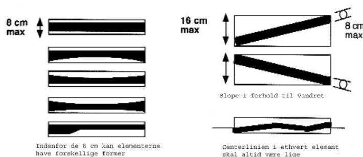
Figur 3 Elementernes dimensioner 1
